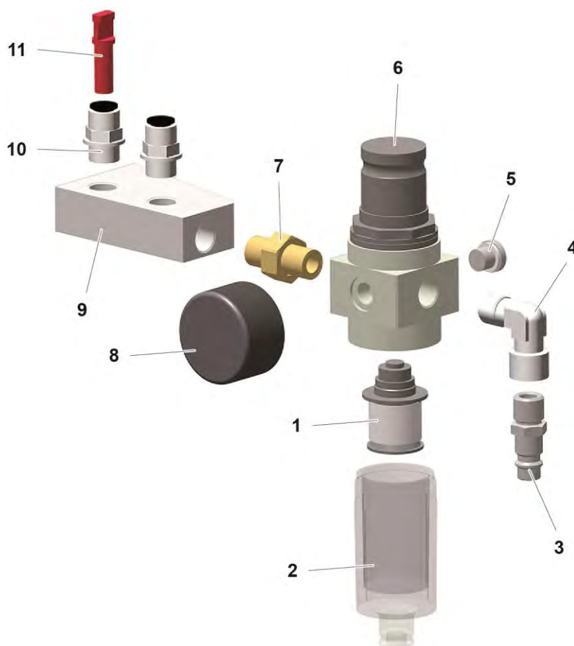
Fig. 13 : Groupe pneumatique
